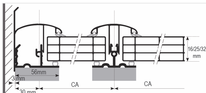
Therm - Mètre de profil mural PVC
